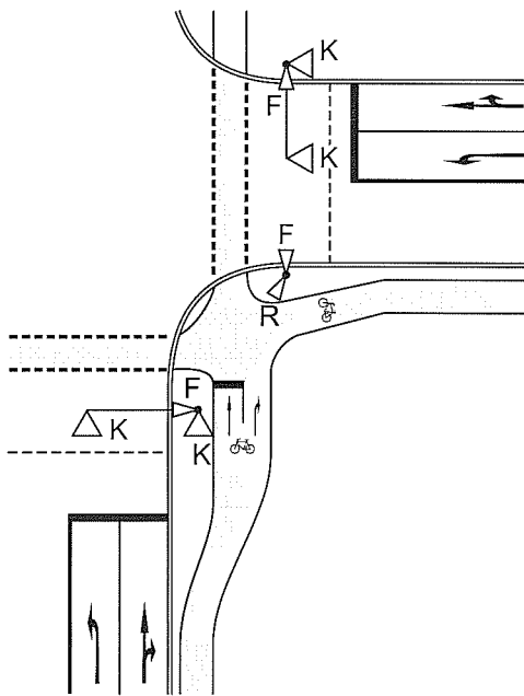
Bild 47: Freies Rechtsabbiegen für den Radverkehr (mit gesonderter Signalisierung des geradeaus fahrenden Radverkehrs)
