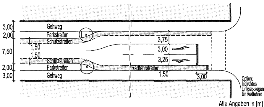
Bild 45: Vorgezogene Haltlinie im Zuge eines Radfahrstreifens
